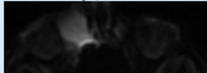
Diffusion (b1000)
